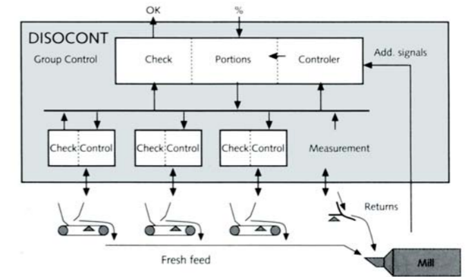
5 Regelung von Kugelumlaufmühlen 5 Control of closed-circuit ball mills
