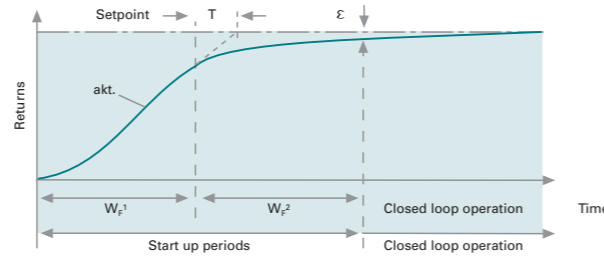
4 Anfahrautomatik 4 Automatic starting system
