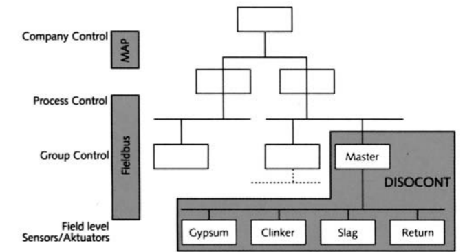
8 Hierarchischer Aufbau der Unternehmensautomatisierung 8 Hierarchical structure of factory automation
